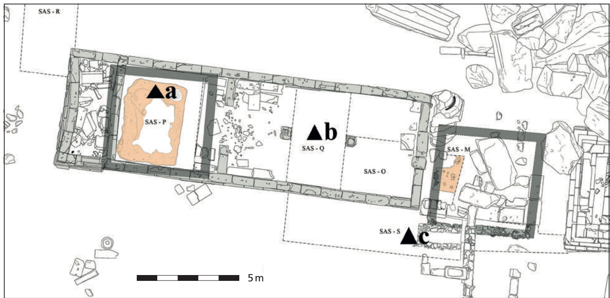
Fig. 2 Pianta del Tempio R, con indicazione delle fondazioni, pavimento, e dimensioni ricostruite delle prime strutture (EB I-II): a indicazione del punto di rinvenimento della cuspidi di lancia in ferro M15.10. – b delle lame in ferro M17.65-67. – c del palco di corna di cervo rosso cons19.142. – (Rilievo M. Limoncelli / F. Pisciotta; © Institute of Fine Arts-NYU).
