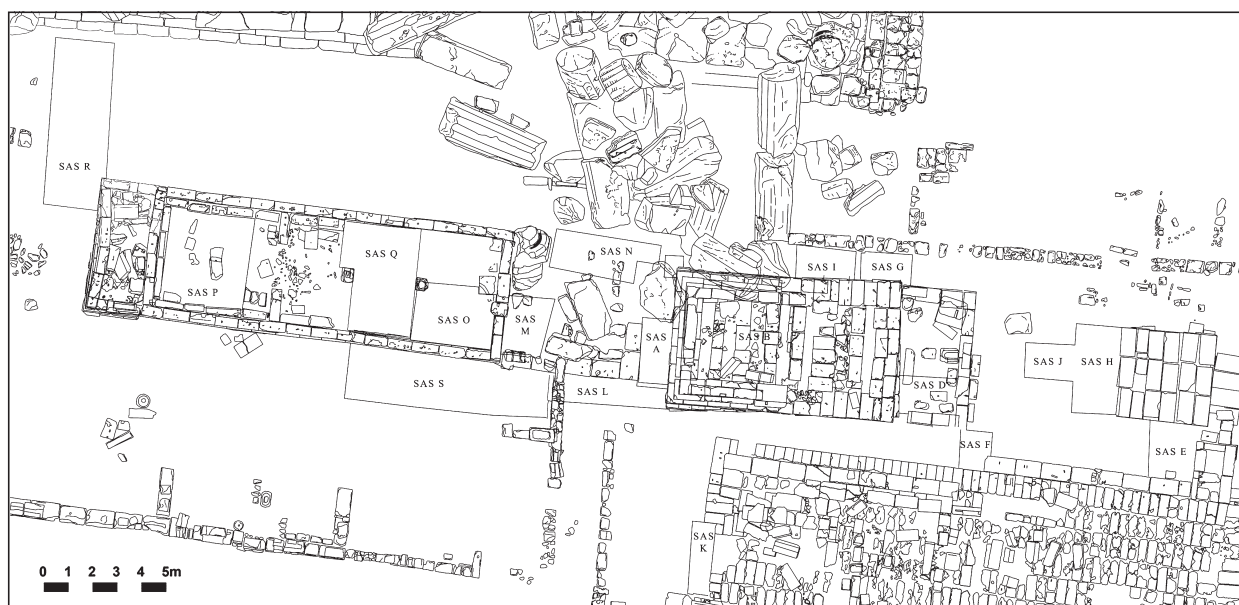
Fig. 1 Pianta del settore meridionale del grande santuario urbano di Selinunte, con indicazione della posizione dei SAS A-S. – (Rilievo M. Limoncelli / F. Pisciotta / D. Scahill; © Institute of Fine Arts-NYU).
