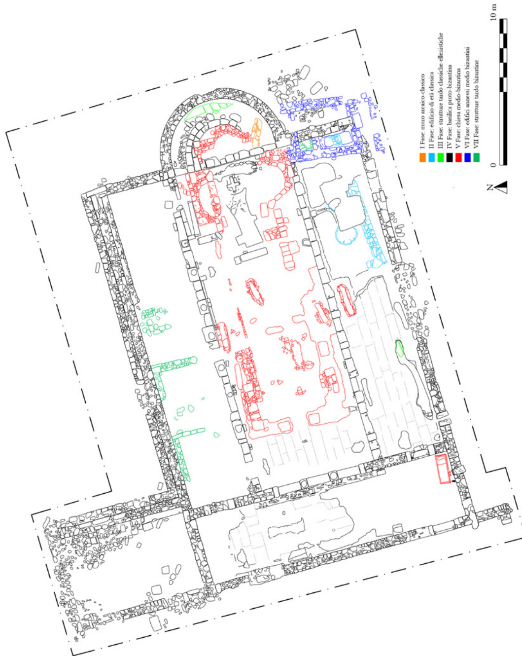
Fig. 3. Efestia. Area del porto orientale. Pianta archeologica della basilica proto-bizantina e delle fasi preesistenti e successive. Scavi 2021 (© Archivio disegni SAIA NIG 8111. El. C. De Domenico).
