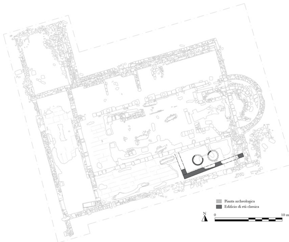
Fig. 21. Efestia. Area del porto orientale. Pianta ricostruttiva dell'edificio di età classica, individuato sotto le strutture della navata S (© Archivio disegni SAIA NIG. 8355. El. C. De Domenico, con aggiornamenti di C. Mendolia).
