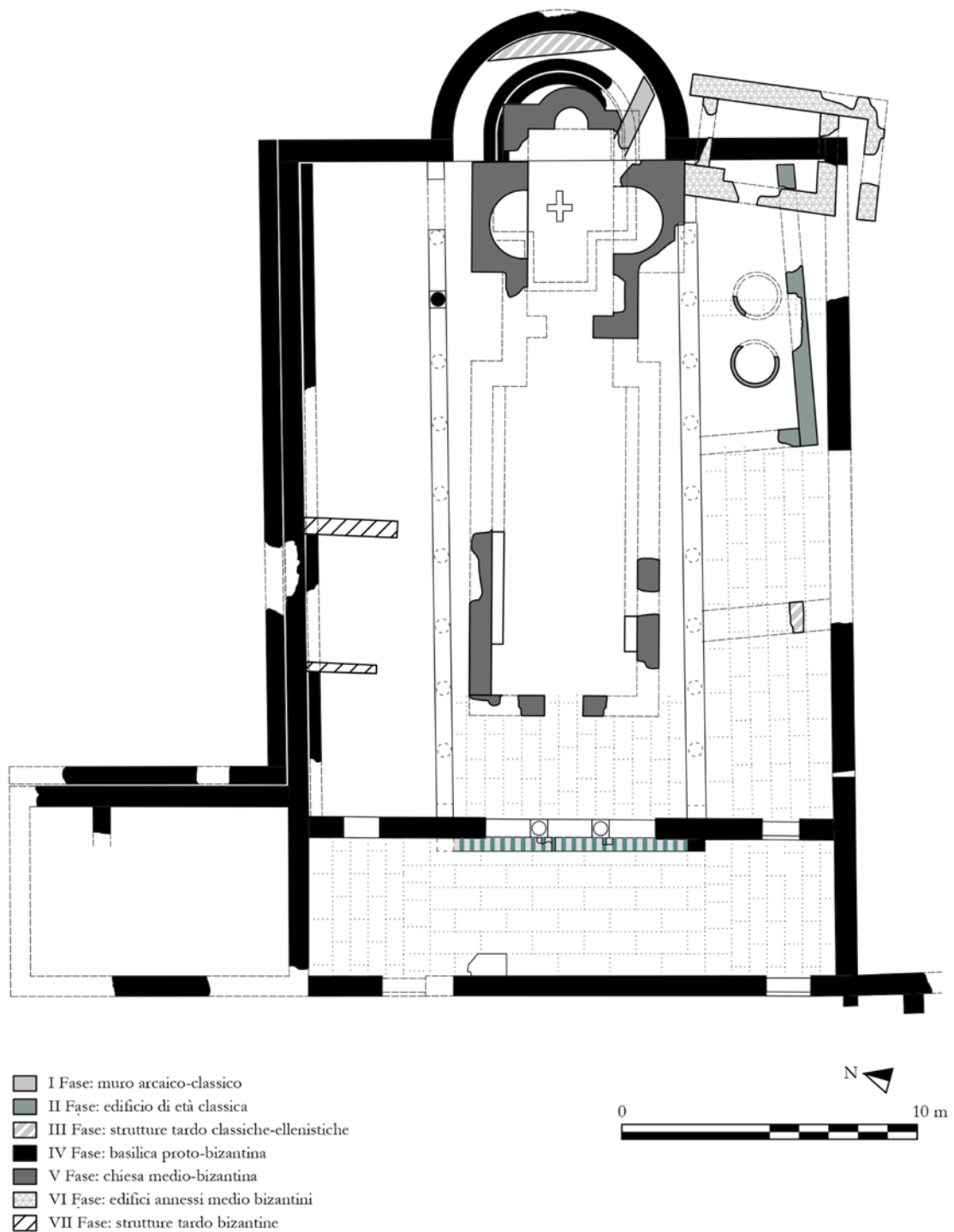
Fig. 20. Efestia. Area del porto orientale. Pianta ricostruttiva della basilica proto-bizantina e delle fasi preesistenti e successive. Scavi 2021 (© Archivio disegni SAIA NIG.8112. El. C. De Domenico, con aggiornamenti di C. Mendolia).
