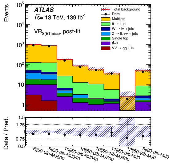
(b) VR_{S(E_T^{miss})}
