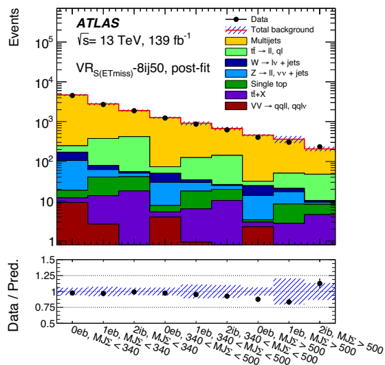
(b) VR_{S(E_T^{miss})}
