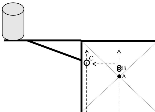
Figura 3. Il Centro di Gravità (CG) idealmente posto a metà della lunghezza delle gambe del tavolo (punto "A") è in realtà spostato più in alto (punto "B") in funzione del peso del ripiano. La presenza di una ribaltina o prolunga del tavolo, con poggiato un oggetto pesante, sposta a sinistra il punto di gravità (punto "C")
