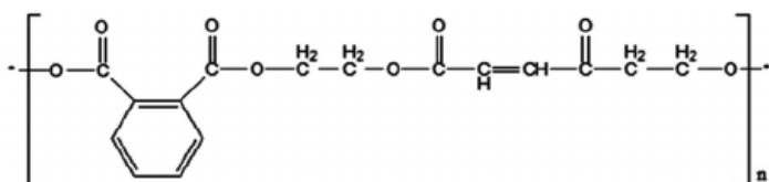
Formula generica di resine poliesteri insature
