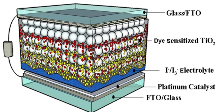
Fig. 5 - Schema di una Dye-Sensitized Solar Cell (DSSC)
