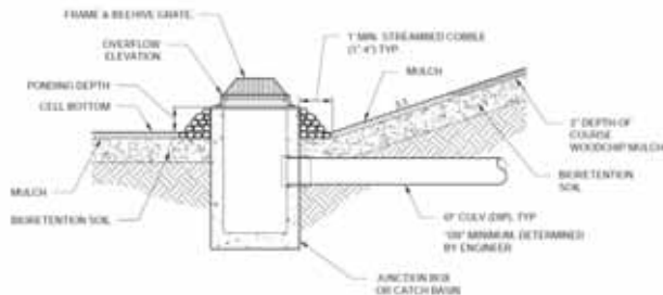
Fig. 1.8: schema di troppopieno.
