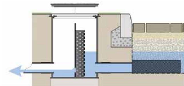
Fig. 1.2: schema di riduttore di flusso.
