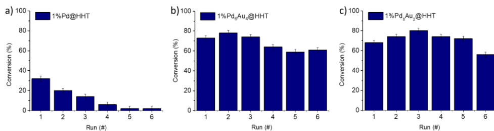
Figure 7. Recycling tests a) monometallic 1%Pd@HHT b) 1%Pd 6 Au 4 @HHT c) 1%Pd 6 Au 2 @HHT.
