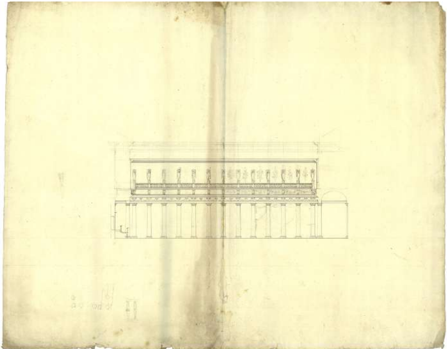
6. Luigi Canonica, Scuderie di Villa Reale, Monza, prospetto sud, [1807].
