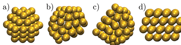
Fig. 1 The structure of some Au 55 isomers from Table 1: (a) Cub; (b) 5; (c) 8; (d) 1.
