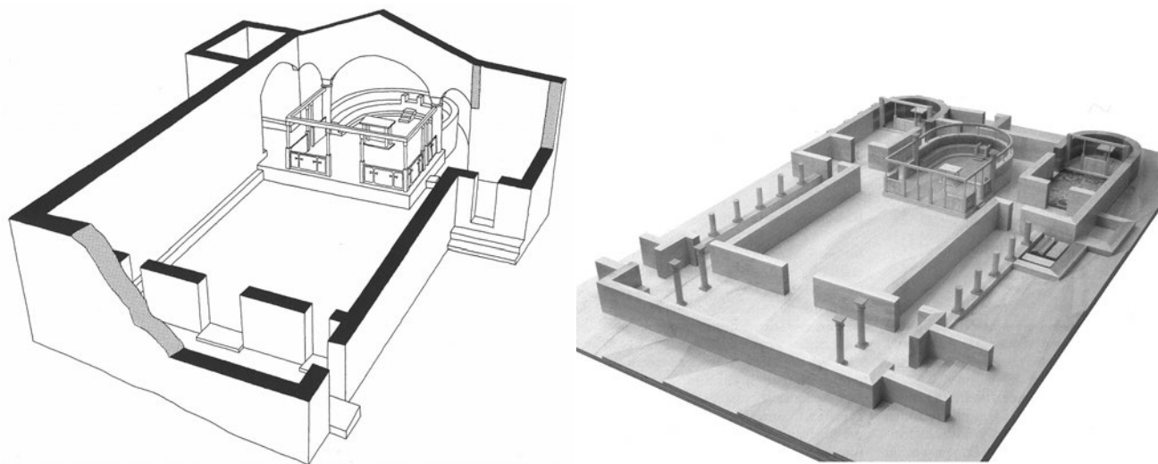
Fig. 3. Teurnia/Tiburnia, presso l'odierna Sankt Peter in Holz (Carinzia). Restituzione assonometrica della Bischofskirche e modello della Friedhofskirche, con bema, synthronos e cancelli (da GLASER 2003a).
