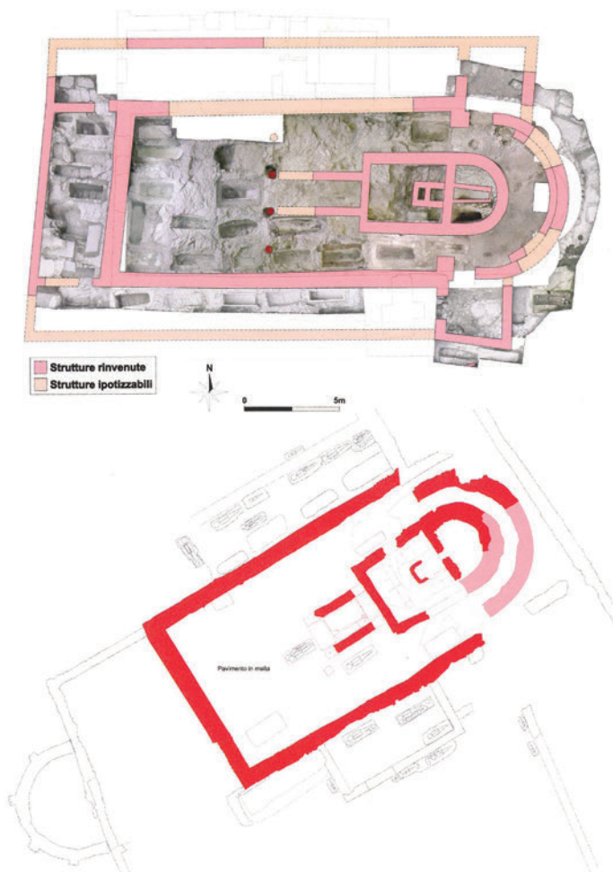
Fig. 4. Bema absidato con solea: Sirmione, San Pietro in Marvinas; Riva del Garda, San Cassiano (da BROGIOLO 2011a).
