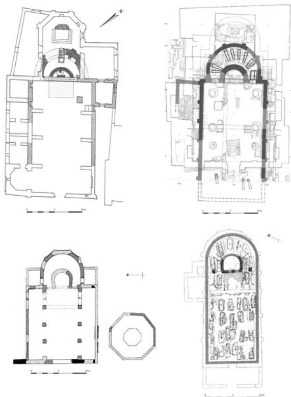
Fig. 2. Planimetrie in scala di quattro chiese di V-VI secolo con bema e synthronos (da scavo). In senso orario da sinistra in alto: Nave (BS), pieve di Santa Maria della Mitria (da BREDA, PARECCINI 2001); Aosta, Santo Stefano (da PERINETTI 2005); Sizzano (NO), pieve di San Vittore (da PEJRANI BARICCO 2003); Gozzano (NO), pieve di San Lorenzo (da PEJRANI BARICCO 2003).
