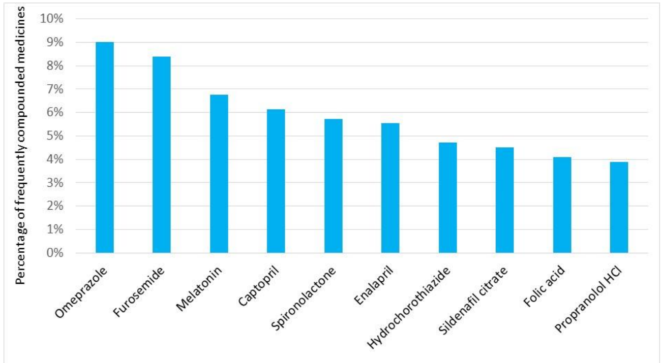
Fig. 2e South America
