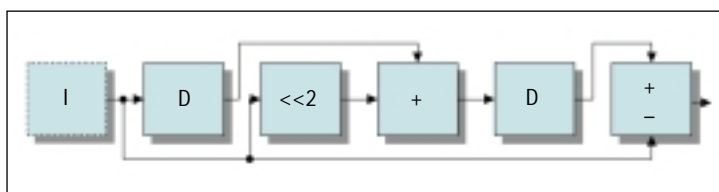
FIGURA 3 Diagramma schematico di un esempio di circuito ottenuto per composizione di 6 operazioni primitive
