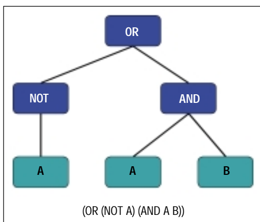
FIGURA 1 Un esempio di programma LISP con il suo albero di parsing associato
